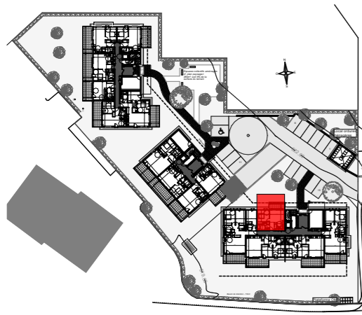
Plan masse
